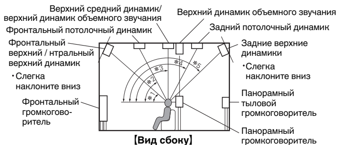
[Вид сбоку]
