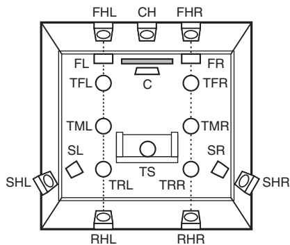
【顶视图】
