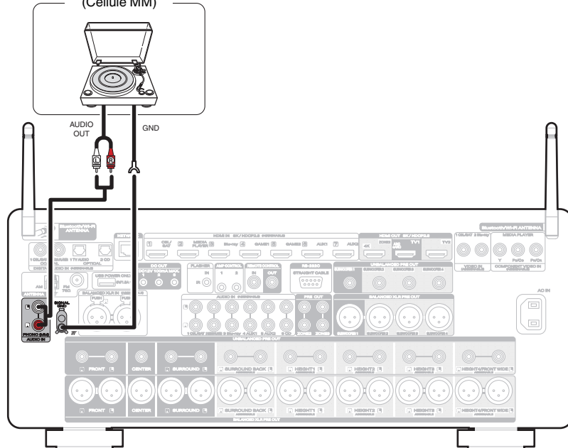
Lecteur d'enregistrement (Cellule MM)
