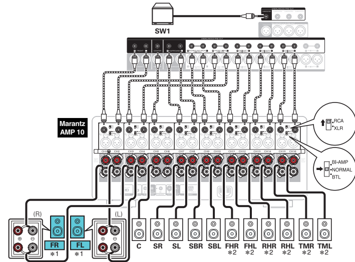
[Anschlussbeispiel] UNBALANCED RCA-Anschluss
