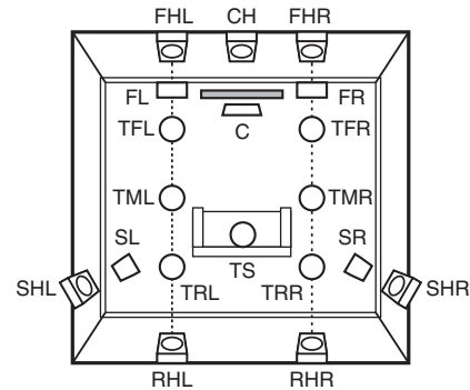
[Draufsicht]
