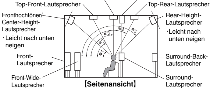
[Seitenansicht]
