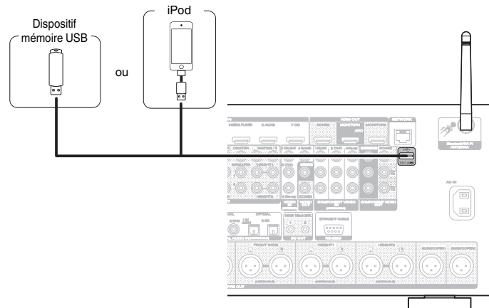
[Panneau arrière]
