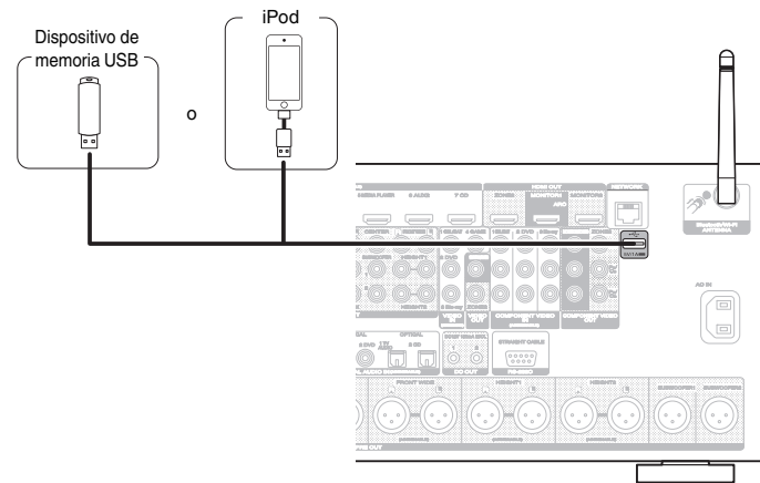
【Panel trasero】
