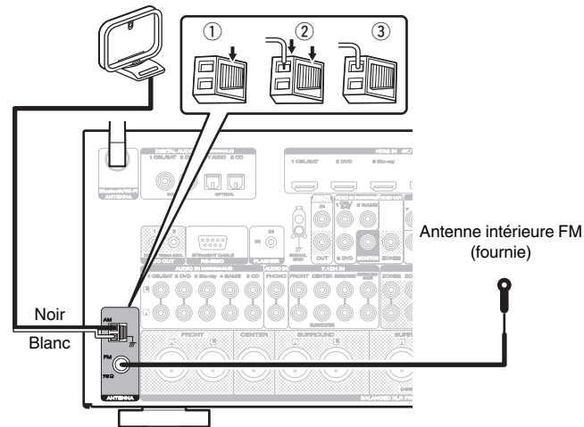
Antenne à boucle AM (fournie)
